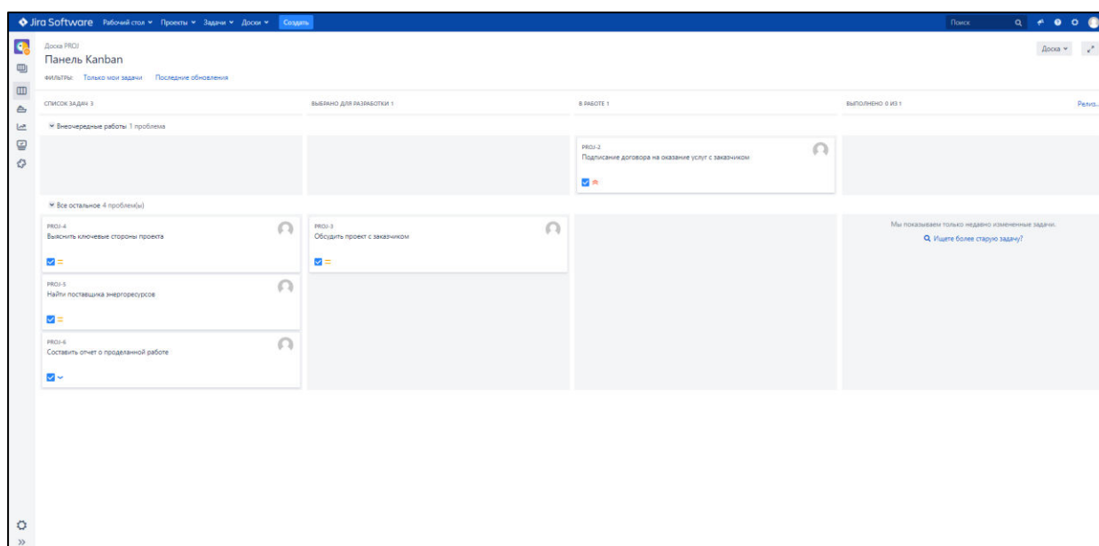
Рисунок 4 – Панель Kanban
